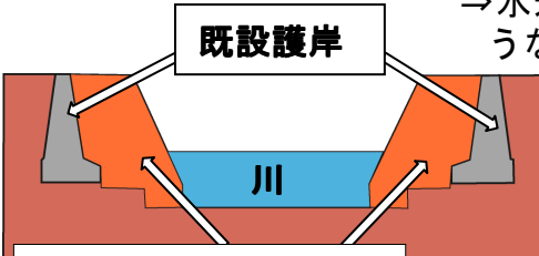
計画護岸(親水護岸)
